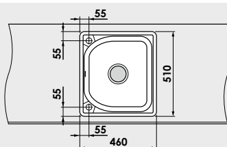
Монтажен отвор
