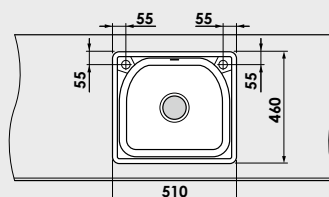
Монтажен отвор
