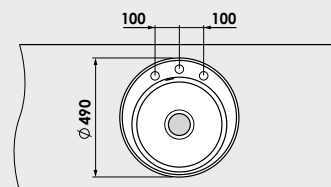
Монтажен отвор
