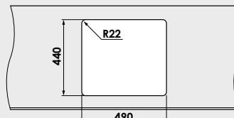
База шкаф
